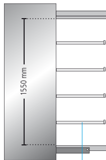
Je Auszug 4 Verstellböden Nutzmass je Verstellboden: B 291/210 x T 584 x H 25
